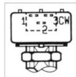
4 Raster: 2.5 mm Ansicht: von oben 4 grid: 2.5 mm top view
