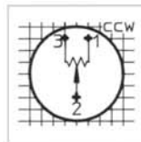
3 Raster: 2.5 mm Ansicht: von oben 3 grid: 2.5 mm top view
