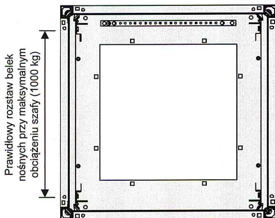
Szafa o szerokości 600 mm
