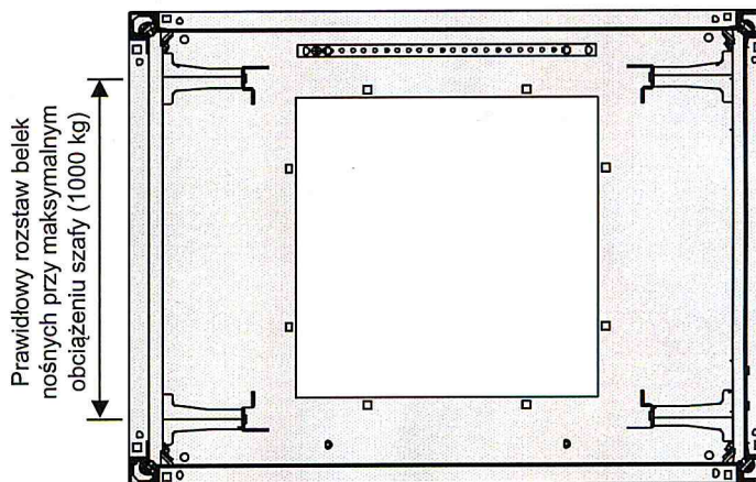
Szafa o szerokości 800 mm
