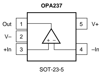
SOT-23-5
