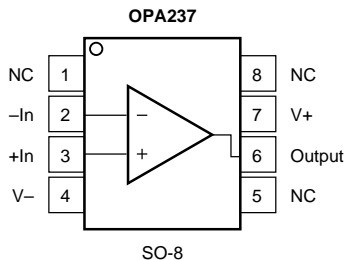
SO-8
