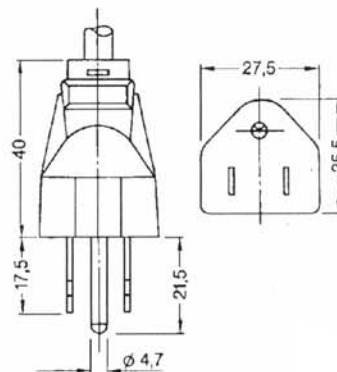
UL-/CSA-Stecker
