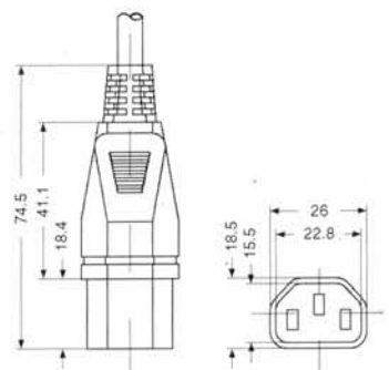
Kaltgerätesteckdose
