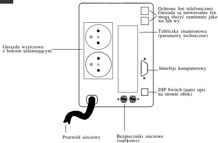
Widok tyłu zasilacza.
