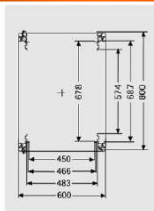
• widok z góry na ramę W x G = 600 x 800
