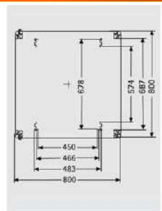
• widok z góry na ramę W x G = 800 x 800
