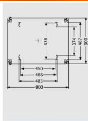
• widok z góry na ramę W x G = 800 x 600
