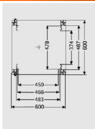
• widok z góry na ramę W x G = 600 x 600
