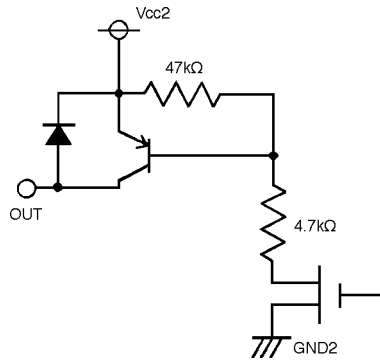
Fig. 7b - Pin 40
