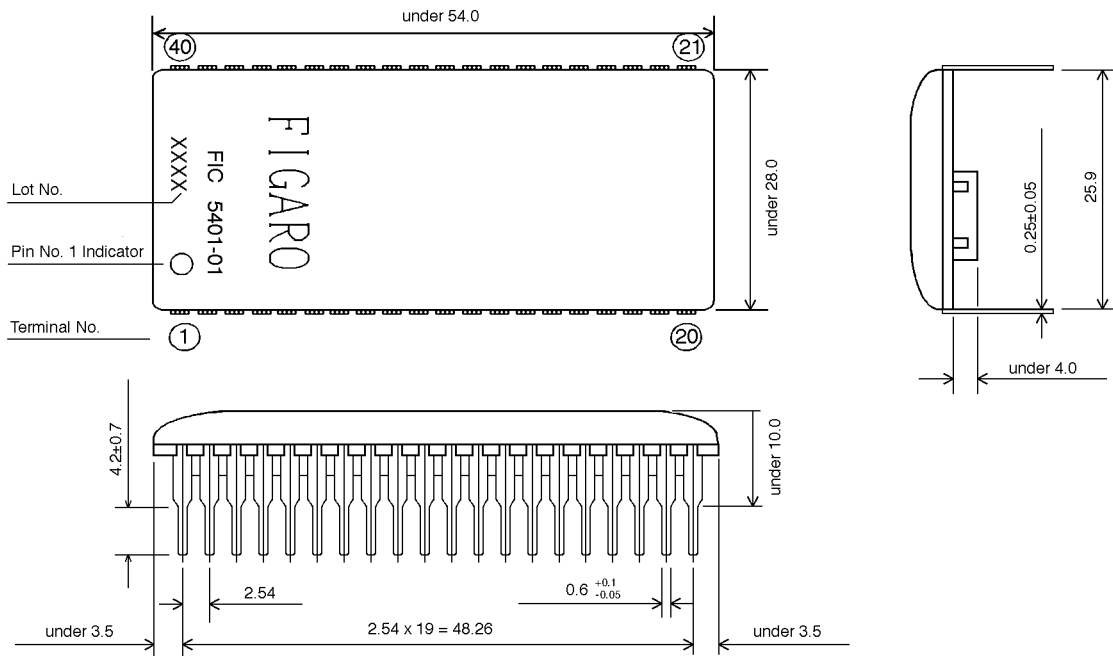
Fig. 6 - FIC-5401 Dimensions (u/m=mm)
